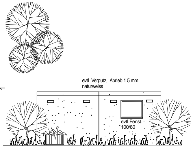
Rückansicht
