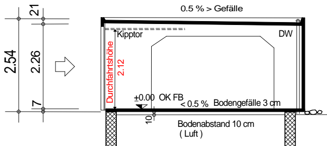
Längsschnitt
