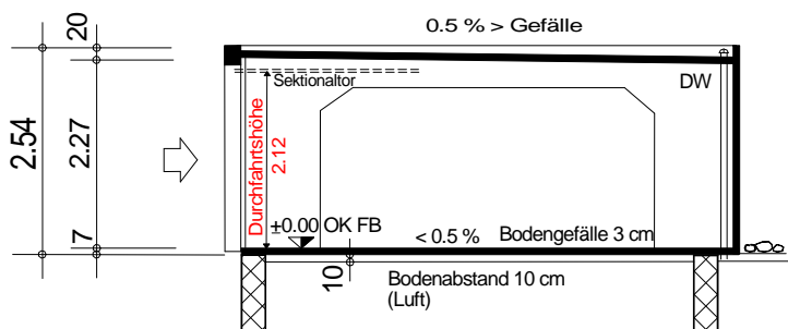
Längsschnitt
