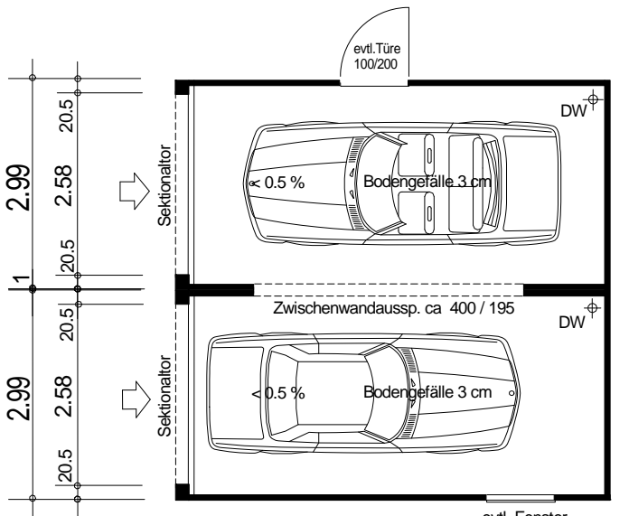
Grundriss
