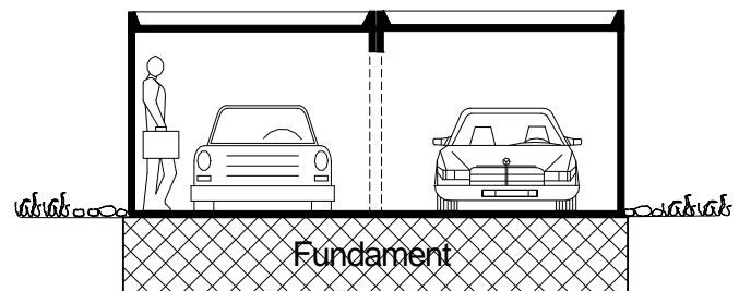
Querschnitt
