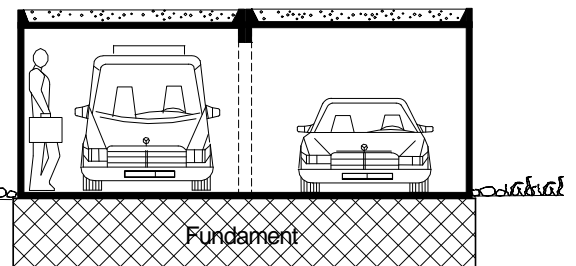
Querschnitt
