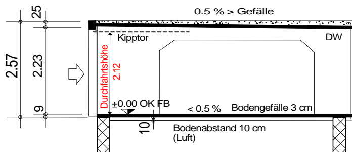
Längsschnitt
