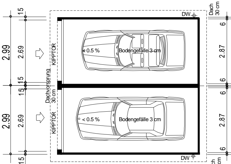
Grundriss
