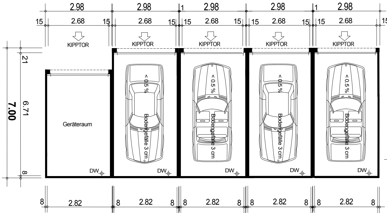
Grundriss
