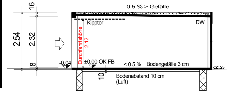
Längsschnitt
