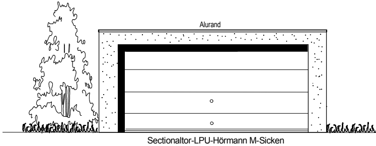
Vorderansicht
