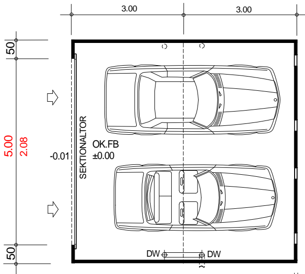
Grundriss
