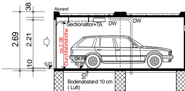
Längsschnitt
