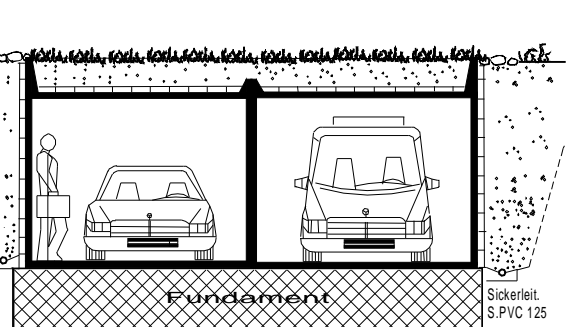
Querschnitt
