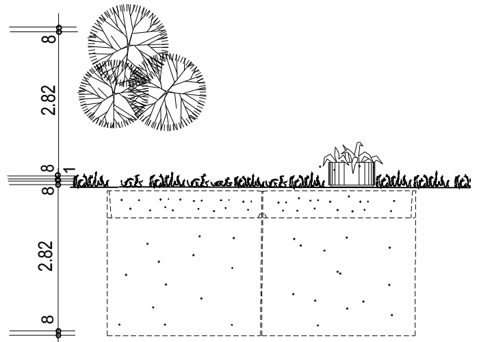
Rückansicht
