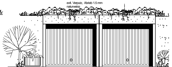
Vorderansicht
