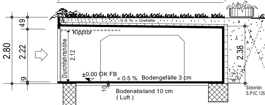
Längsschnitt
