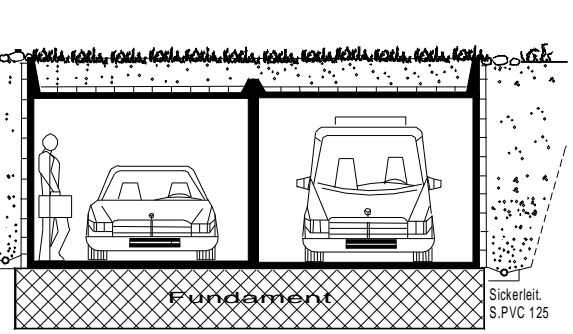
Querschnitt
