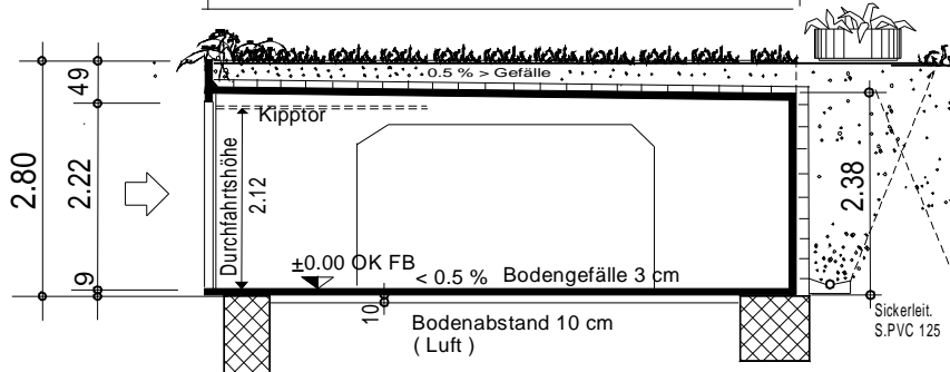
Längsschnitt
