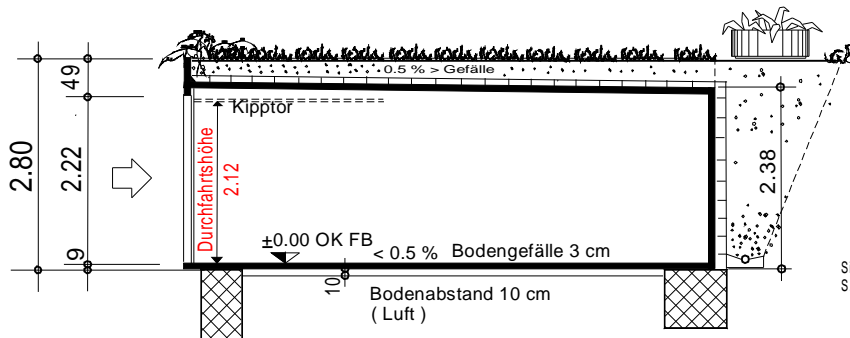
Längsschnitt
