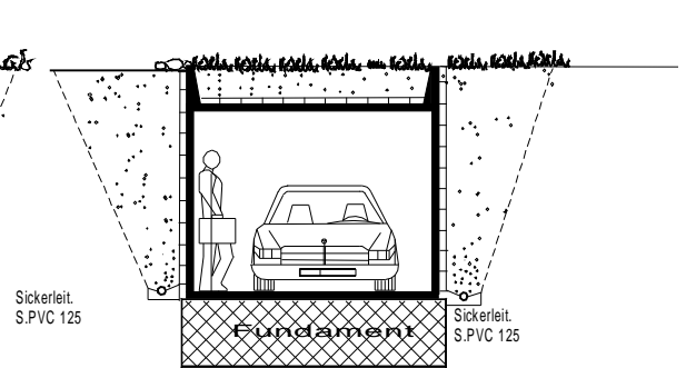
Querschnitt
