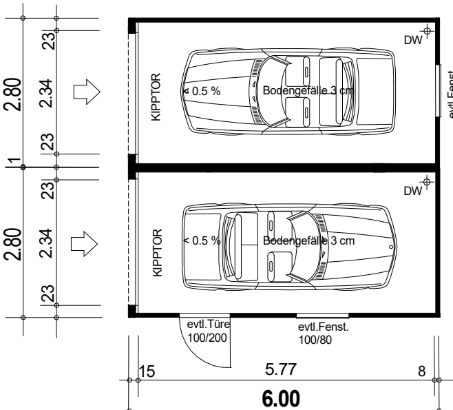
Grundriss
