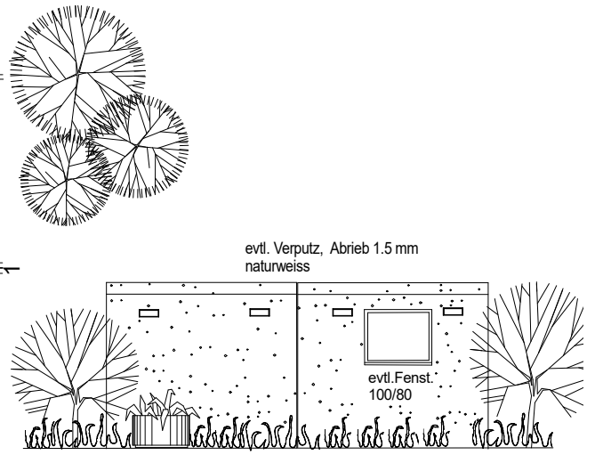
Rückansicht
