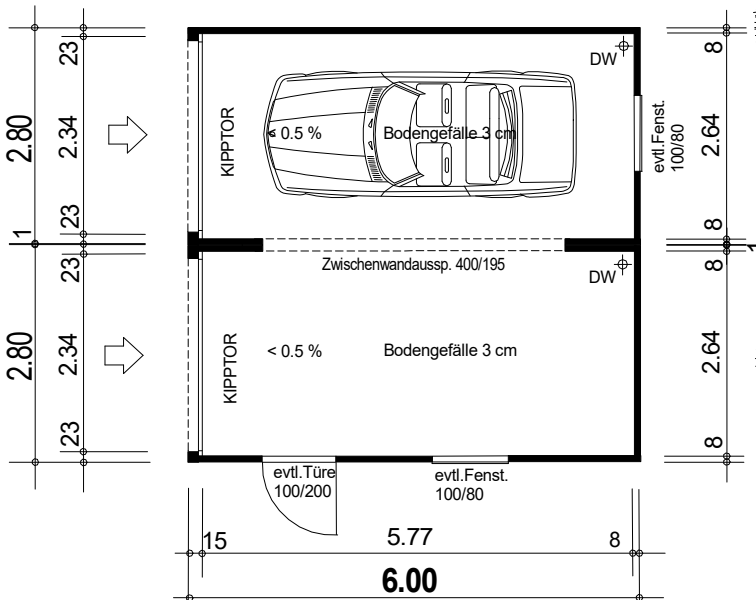
Grundriss
