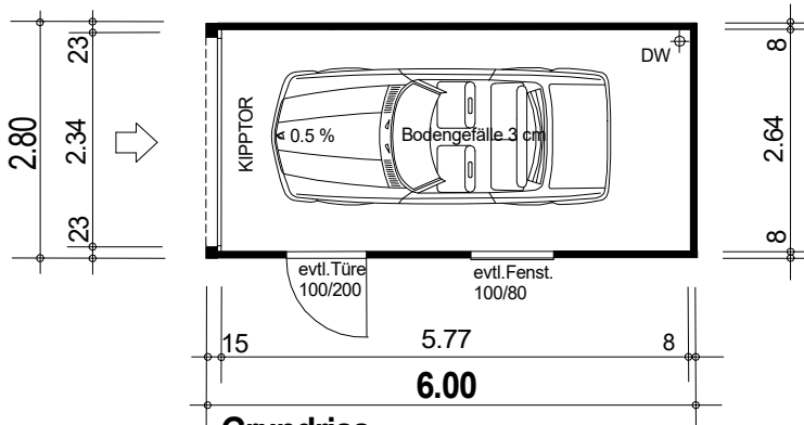
Grundriss
