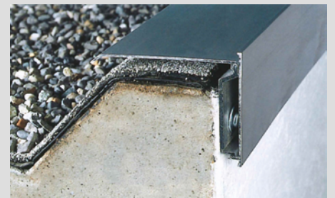
Spenglerblech aus Aluminium. Konkurrenzloser Dachaufbau aus hochwertigen Bitumenschweissbahnen, 4-5 mm stark
