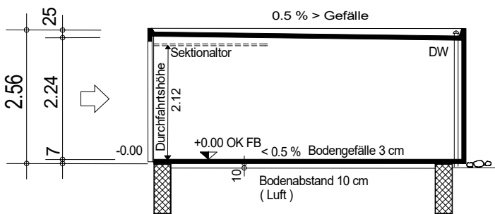
Längsschnitt
