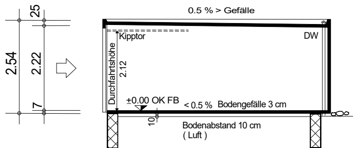
Längsschnitt
