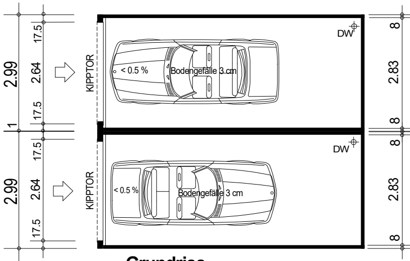
Grundriss
