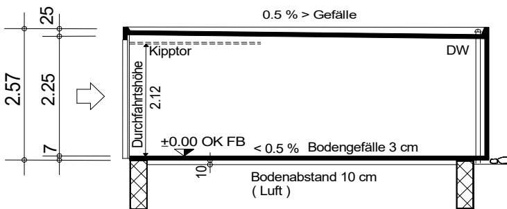
Längsschnitt
