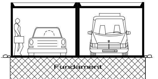
Querschnitt
