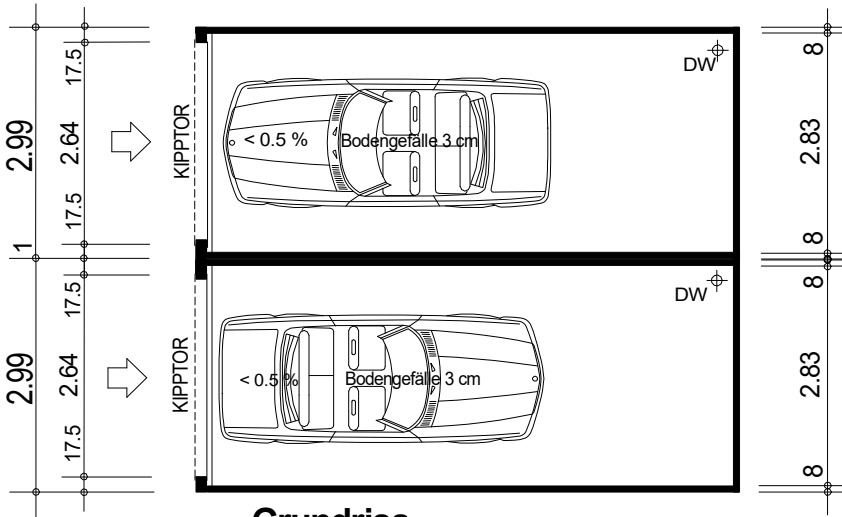
Grundriss
