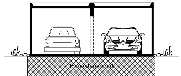
Querschnitt
