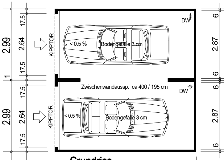
Grundriss
