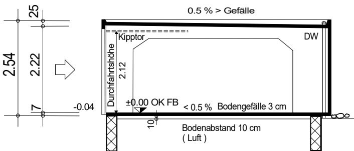
Längsschnitt
