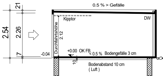
Längsschnitt
