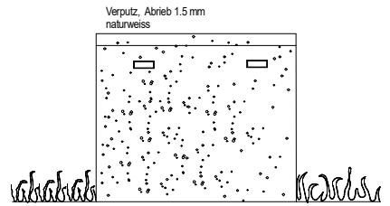
Rückansicht
