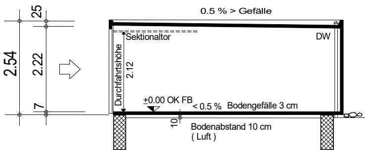
Längsschnitt
