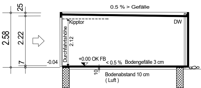
Längsschnitt
