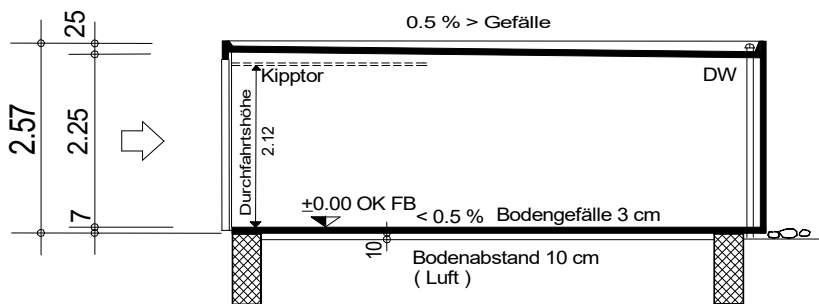
Längsschnitt
