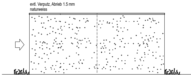
Seitenansicht
