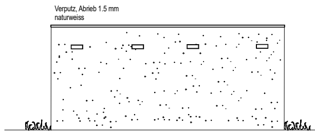
Rückansicht
