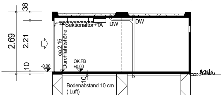
Längsschnitt
