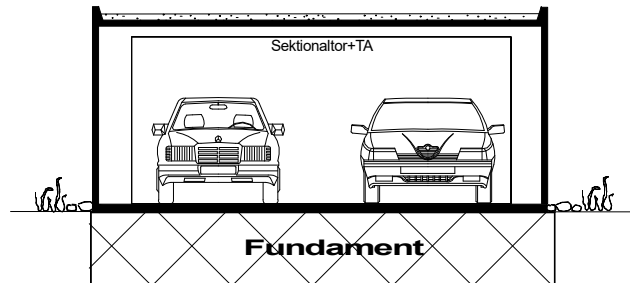
Querschnitt
