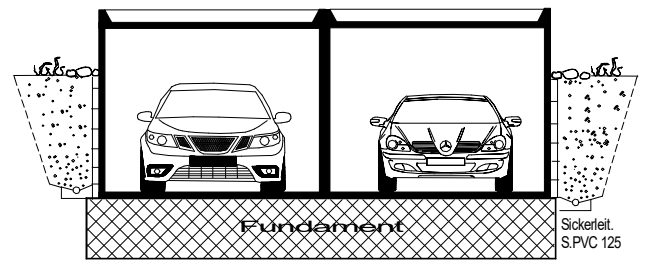
Querschnitt
