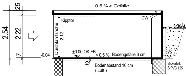
Längsschnitt
