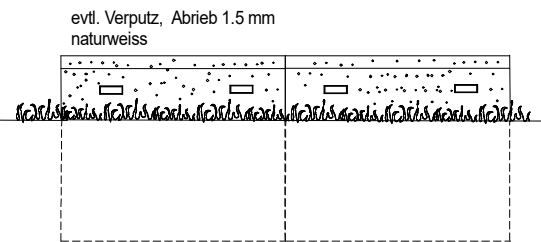
Rückansicht
