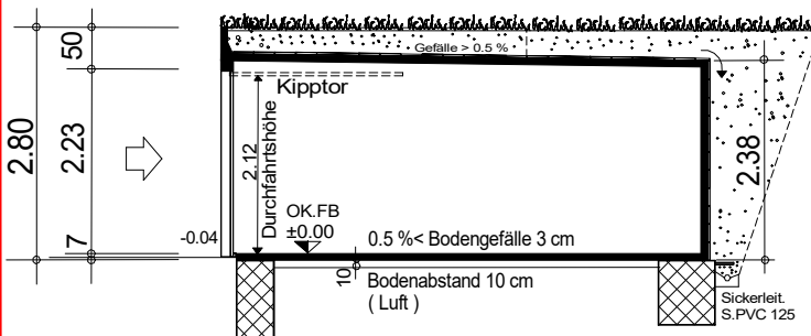
Längsschnitt
