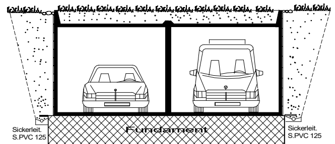
Querschnitt
