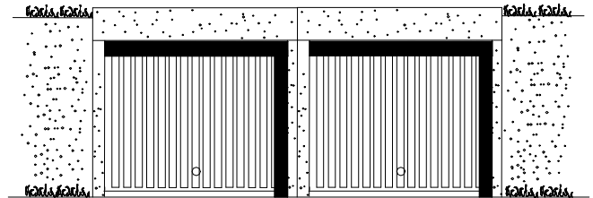
Vorderansicht
