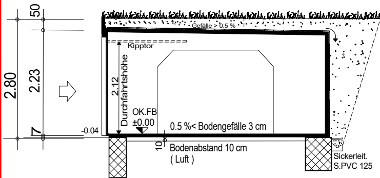
Längsschnitt
