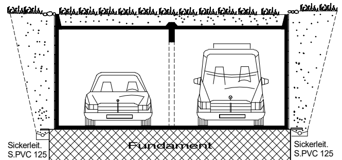
Querschnitt
