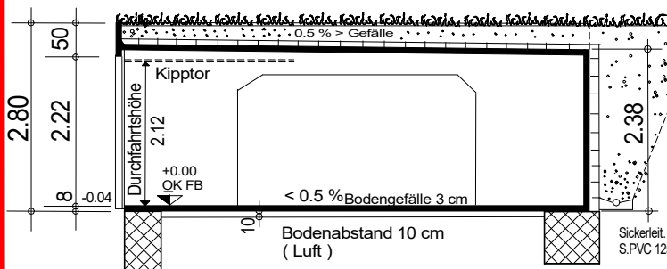
Längsschnitt
