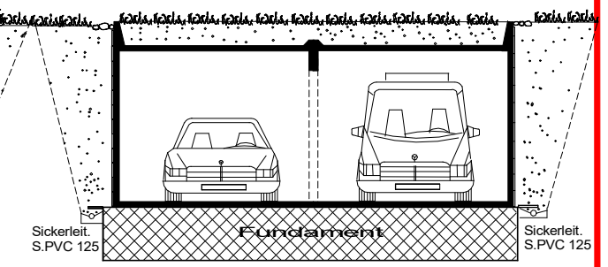
Querschnitt
